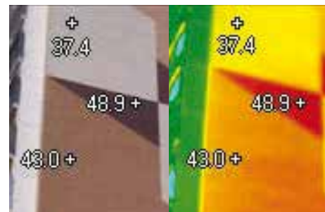
Povrchová teplota na fasáde. Výstup z termokamery 13.00 hod, teplota vzduchu 25 °C.
